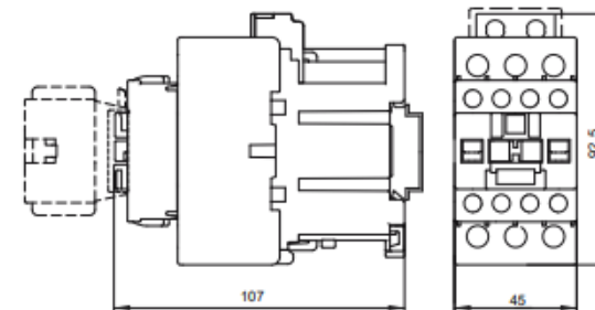
BA47 MC-25~38D (катушка управления DC)
